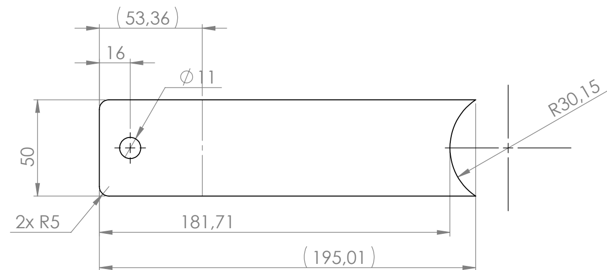
Formatka - na płasko
